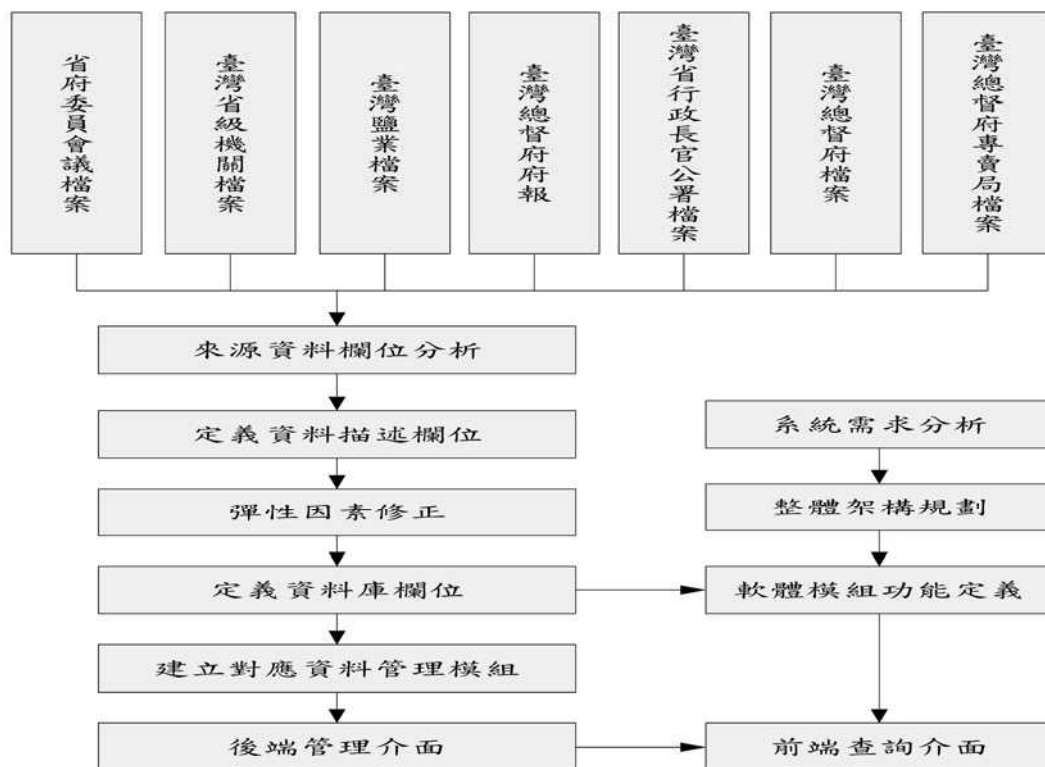
圖 3-3-6：資料庫系統整合作業流程圖
